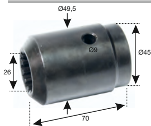
Muffe hinten für Verschleißwelle Allrad 13 Zähne
