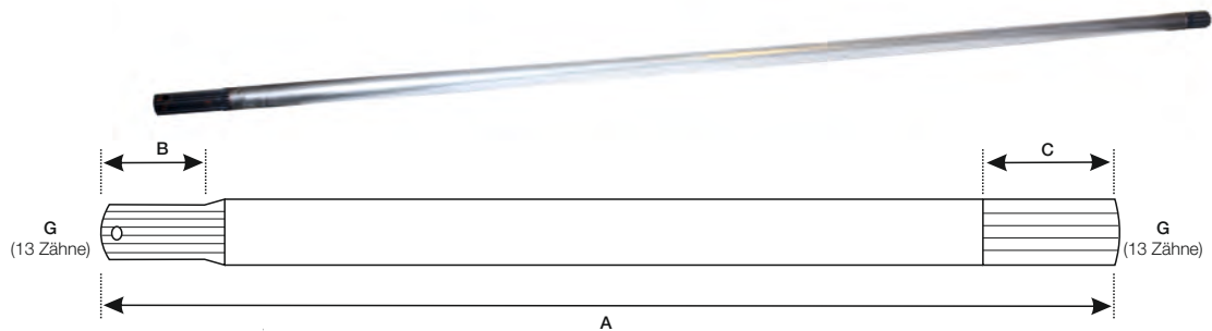
Antriebswelle für Vorderachse Allrad
