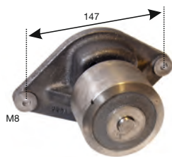
Wasserpumpe für FPT Motor (Fiat Power Train)
